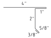
Drip Edge D3
