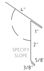
Drip Edge D2
