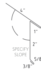
Drip Edge D2
