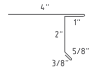
Drip Edge D3
