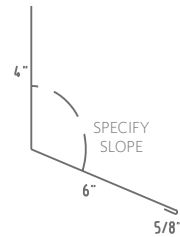
End Wall E1
