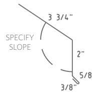
Drip Edge D1
